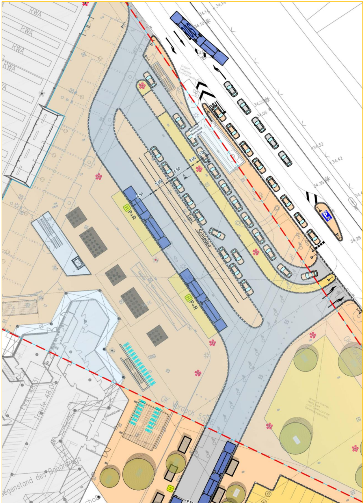
Lageplan Ausschnitt
