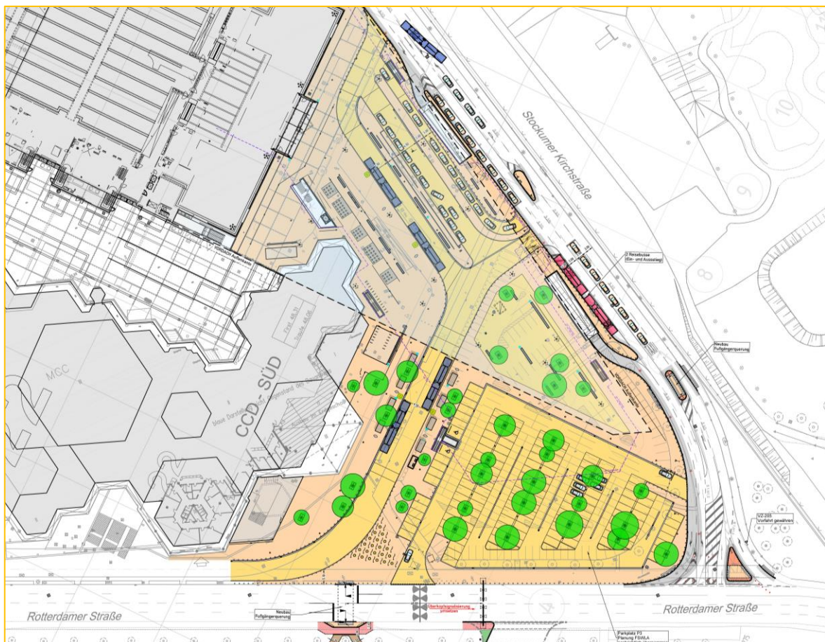
Übersichtslageplan
