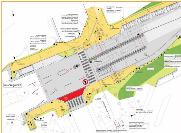
Lageplan Verkehrsanlage
